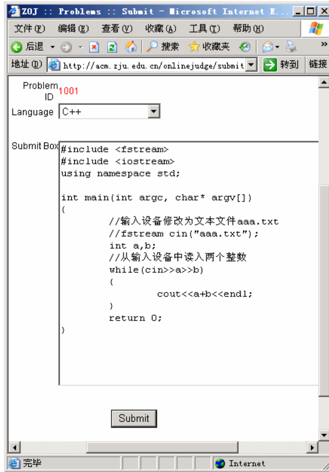
图 1-16 拷贝源代码
