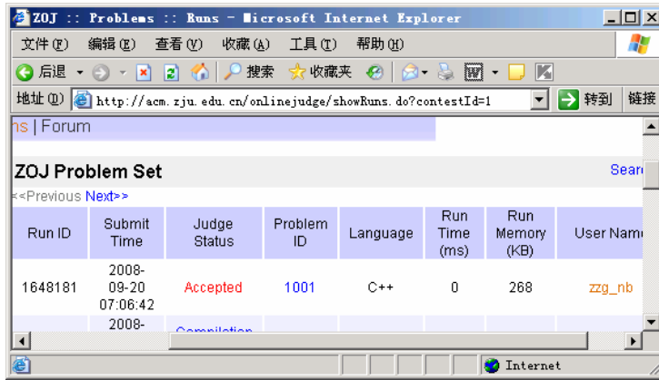
图 1-18 状态页面
