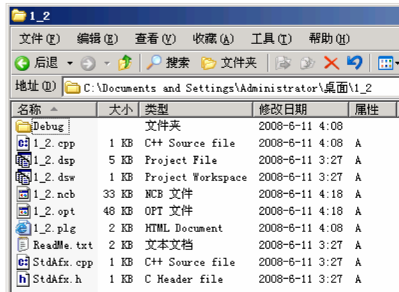
图 1-11 1_2 工程文件
