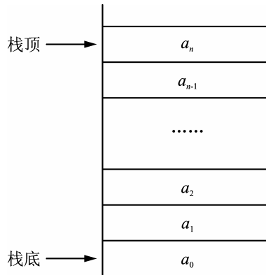
图 2-9 堆栈示意图
